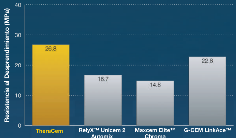
Resistencia al Desprendimiento a la Zirconia
